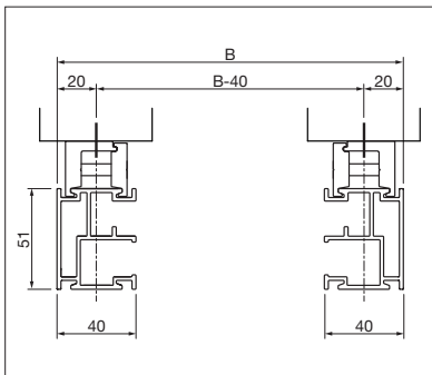
Seitenansicht
