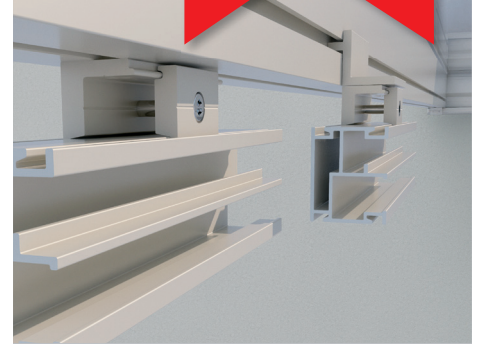
Außenbündige oder eingerückte Montagemöglichkeit
